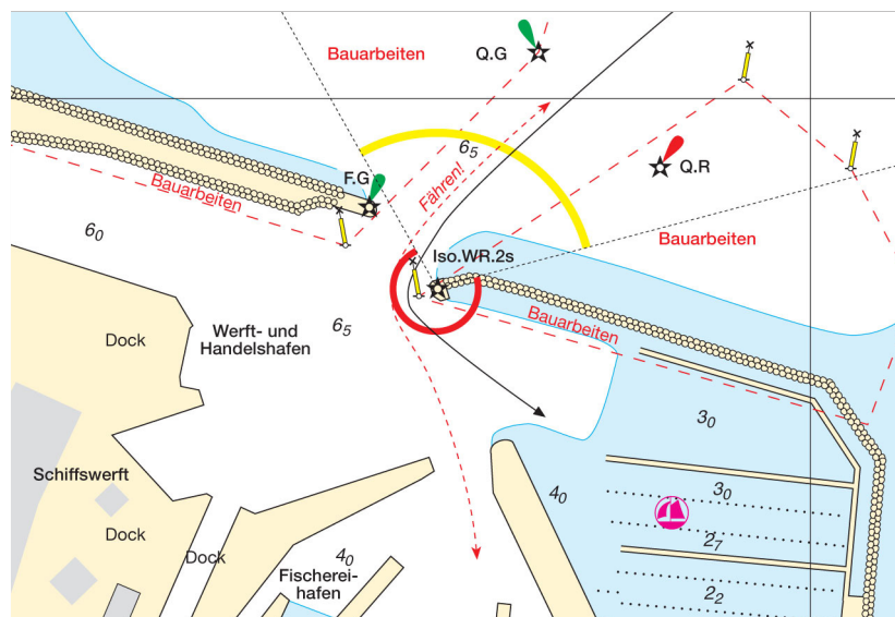
Abbildung 2 - Satz 1 Ausschnitt aus Hafenplan Søby Bauarbeiten Hafenerweiterung/Wellenbrecher
