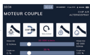
MOTEUR MX À INDUCTION Affichage et présélection de la vitesse des micro-moteurs. Réglage du couple et fonctions auto-reverse et auto-forward. MX INDUCTION MOTOR Micromotor speed display and preselection. Torque adjustment, and auto-reverse and auto-forward functions.
