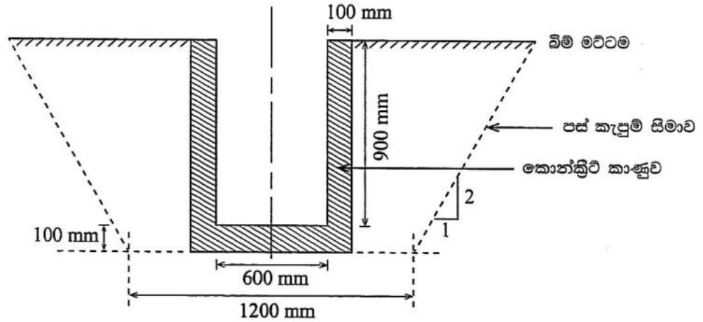
කාණුව සහ පස් කපන සීමාවේ හරස්කඩ පෙනුම
