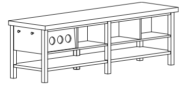
Buffet Table Blue Buffet Table Taupe 3855B01B16 3855B01B15 SP-214.1 SP-214.2 108 x 30 x 34 108 x 30 x 34
