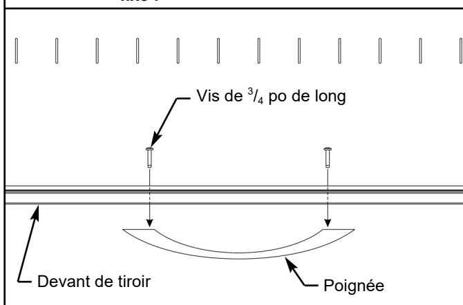
Illustration 3. Installation de la poignée de tiroir à devant fixe :
