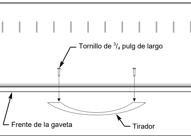
Ilustración 3. Instalación de tirador de gaveta con frente fijo:
