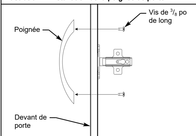
Illustration 4. Installation de la poignée de porte :
