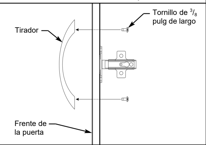
Ilustración 4. Instalación de tirador de puerta:
