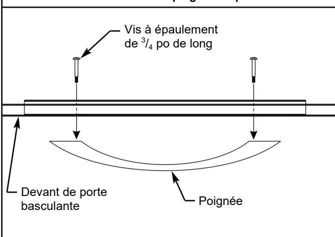
Illustration 2. Installation de la poignée de porte basculante :
