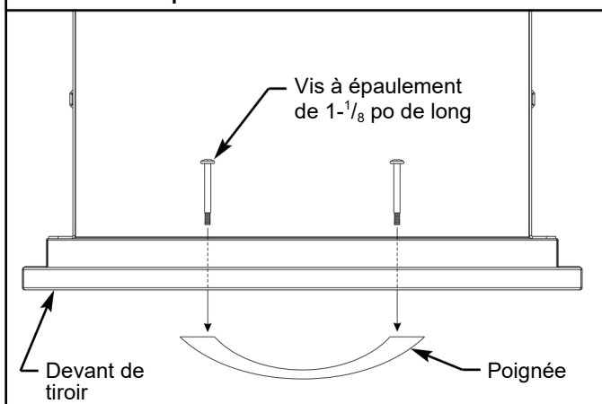
Illustration 1. Installation de la poignée de tiroir du piédestal :
