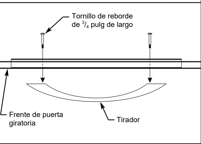
Ilustración 2. Instalación de tirador de puerta giratoria:
