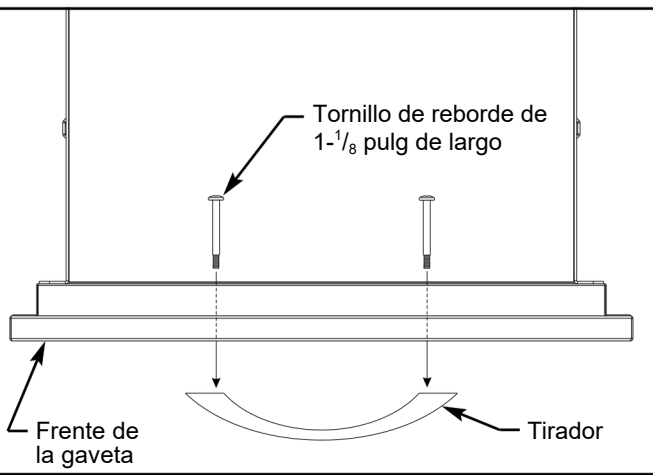
Ilustración 1. Instalación del tirador de gaveta de pedestal:
