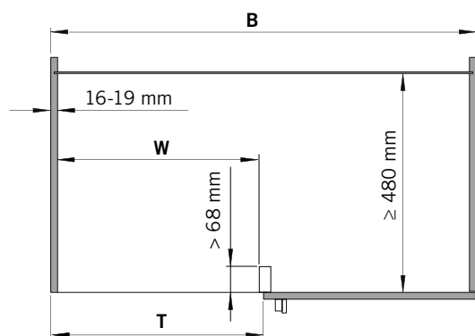
Aufsicht/Top view Ausführung links/Left hand version
