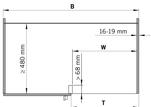
Aufsicht/Top view Ausführung rechts/Right hand version
