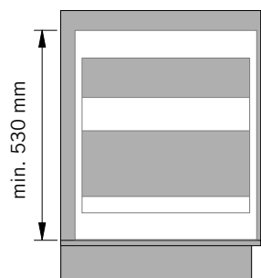
Seitenansicht/Side view
