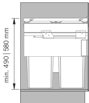
Seitenansicht/Side view
