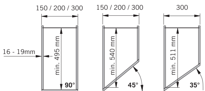
Aufansicht/Top view
