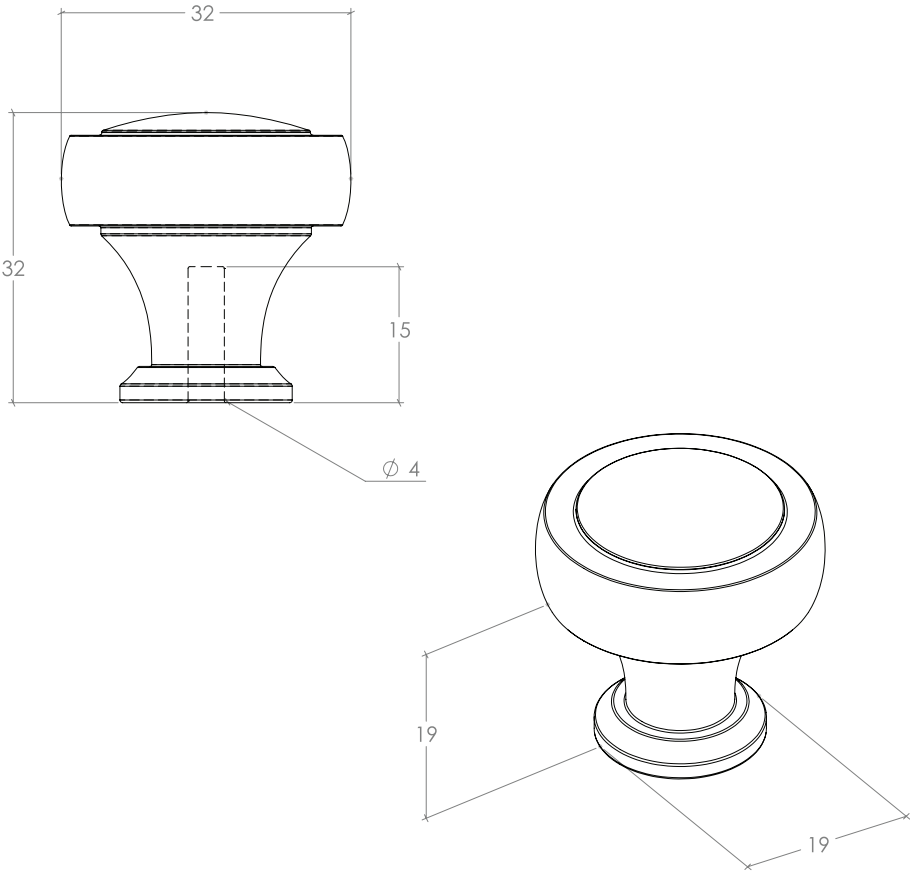
Knob
