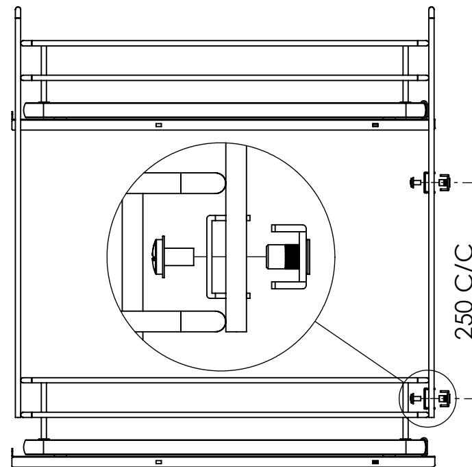
Door Bracket Qty: 02 Nos.
