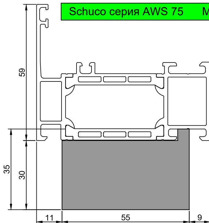
F50-16.07 Тёплый подставочный профиль BLAUGELB 30/35X55X1200MM (Schuco AWS 75)
