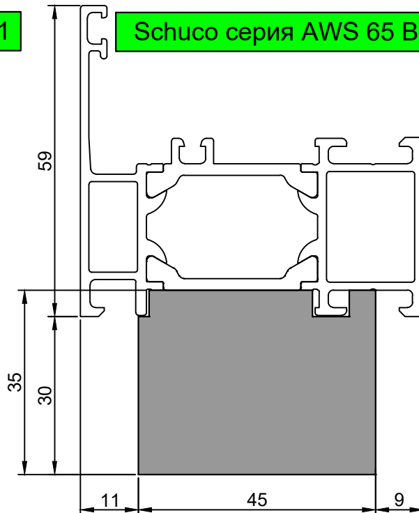
F50-16.04 Тёплый подставочный профиль BLAUGELB 30/35X45X1200MM (Schuco AWS 65 BS)
