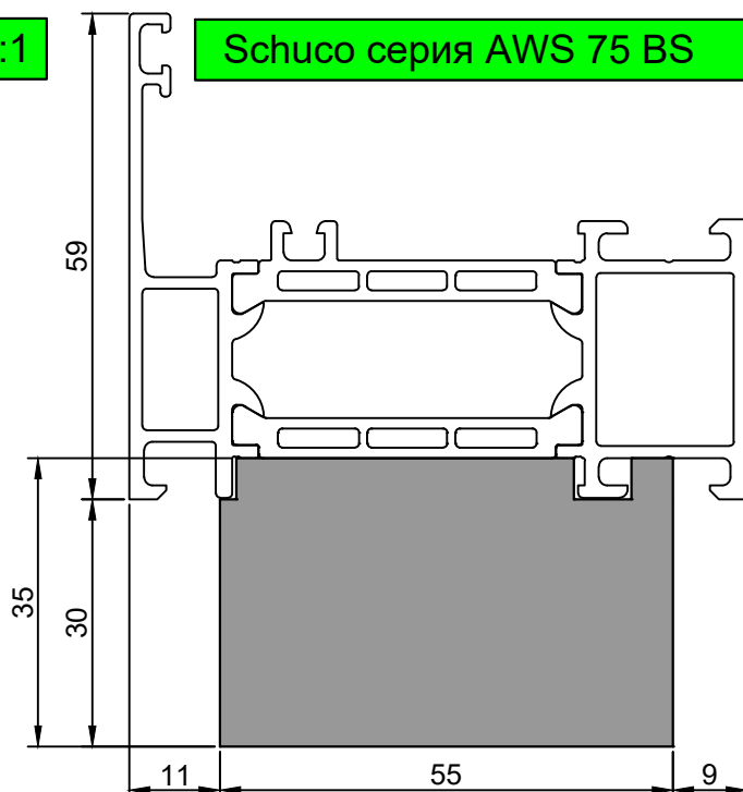
F50-16.08 Тёплый подставочный профиль BLAUGELB 30/35X55X1200MM (Schuco AWS 75 BS)
