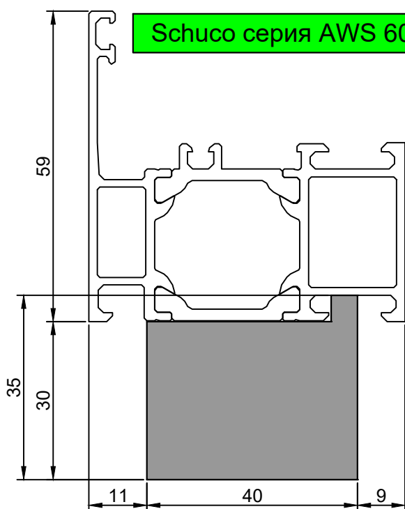
F50-16.01 Тёплый подставочный профиль BLAUGELB 30/35X40X1200MM (Schuco AWS 60)
