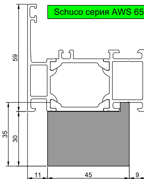
F50-16.03 Тёплый подставочный профиль BLAUGELB 30/35X45X1200MM (Schuco AWS 65)
