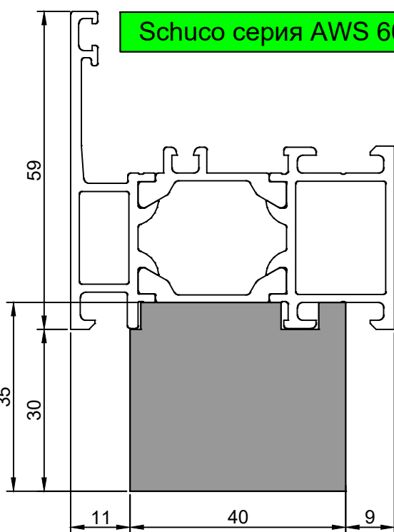
F50-16.02 Тёплый подставочный профиль BLAUGELB 30/35X50X1200MM (Schuco AWS 60 BS)
