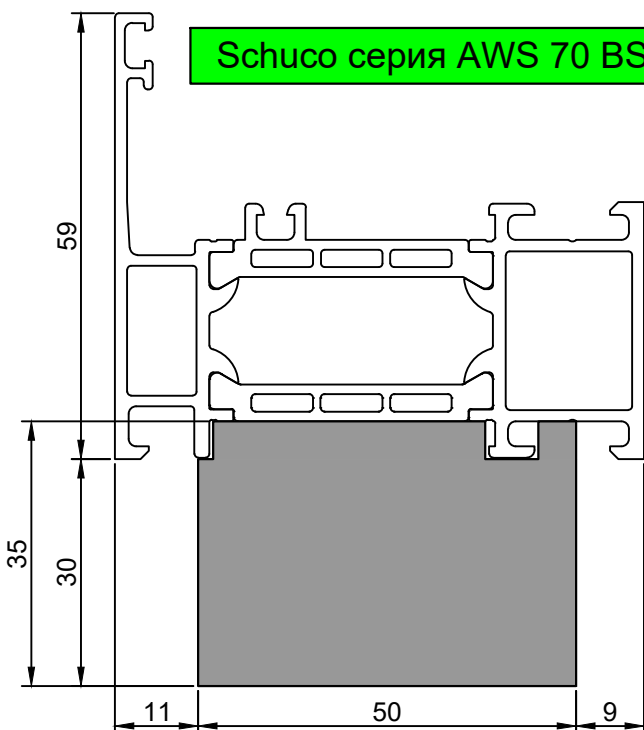
F50-16.06 Тёплый подставочный профиль BLAUGELB 30/35X50X1200MM (Schuco AWS 70 BS)
