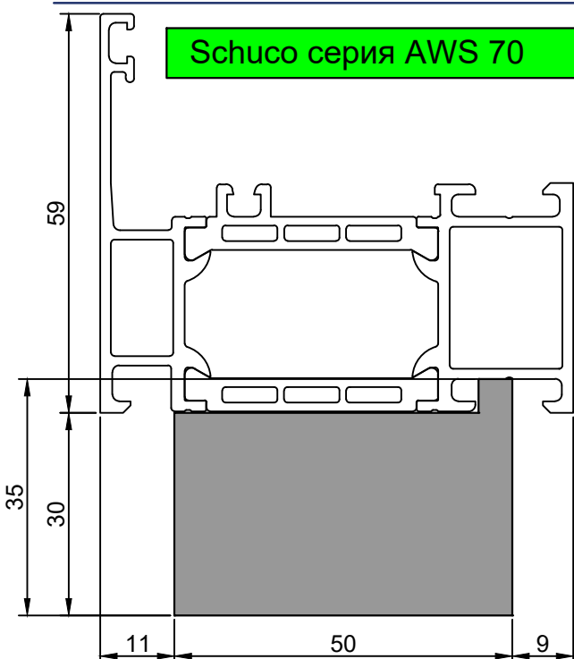
F50-16.05 Тёплый подставочный профиль BLAUGELB 30/35X50X1200MM (Schuco AWS 70)
