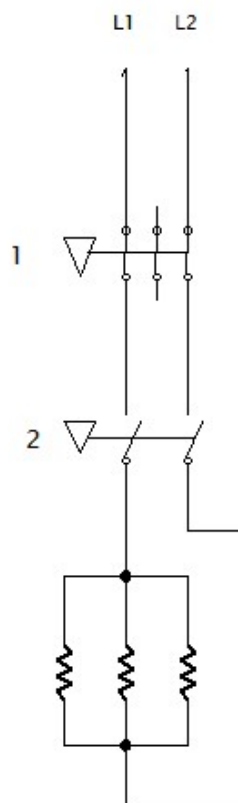
El-skjema 1-fas for inntil 3 kW el-kolbe
