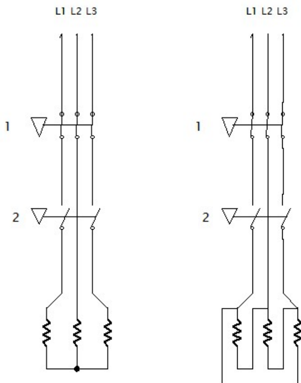
El-skjema 3-fas for inntil 6 kW el-kolbe
