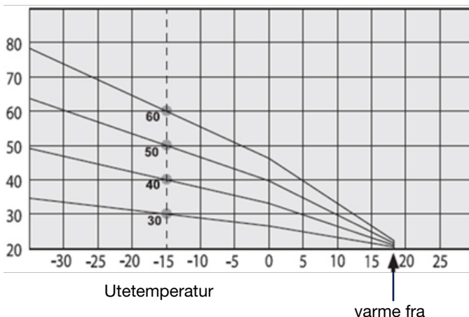
Primær kjeletemperatur
