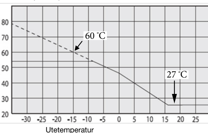
Primær kjeletemperatur
