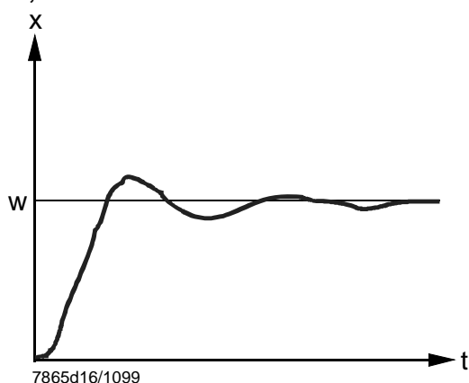
Figura 29: rt, dt insuficiente
