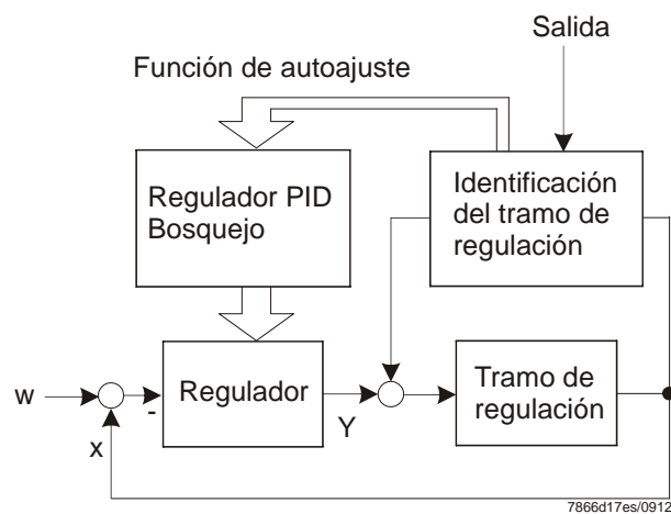
Figura 24: Función de autoajuste en el funcionamiento con carga nominal
