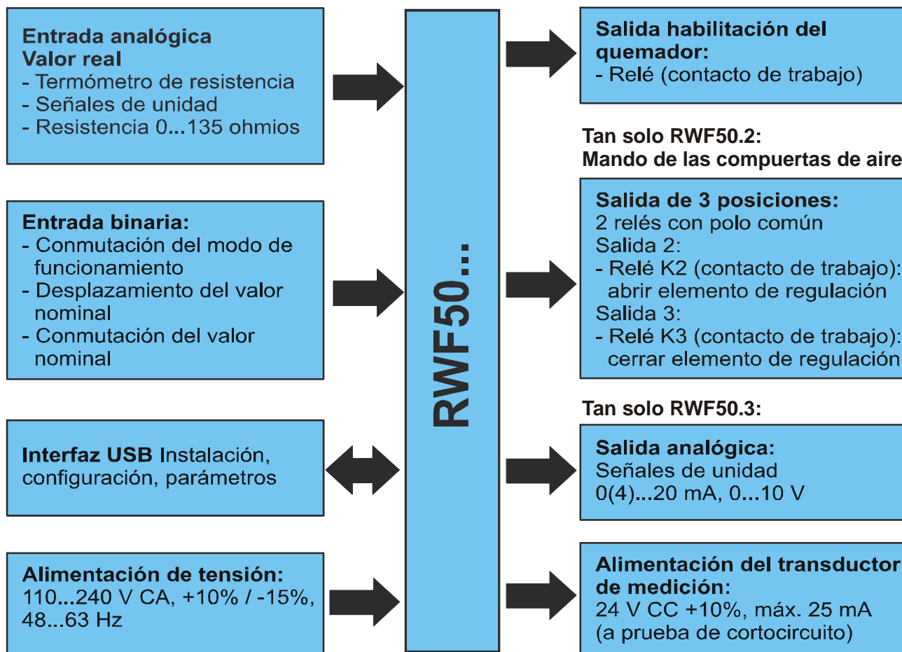
Figura 1: Estructura de bloques
