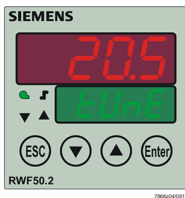
Figura 19: Indicación de la función de autoajuste
