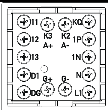
Figura 5: Asignación de terminales
