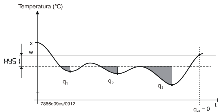
Figura 13: Secuencia de control del umbral de reacción (q)
