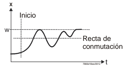
Figura 25: El valor real y el valor nominal están muy alejados entre sí
