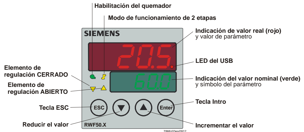
Figura 16: Significado de las indicaciones y de las teclas
