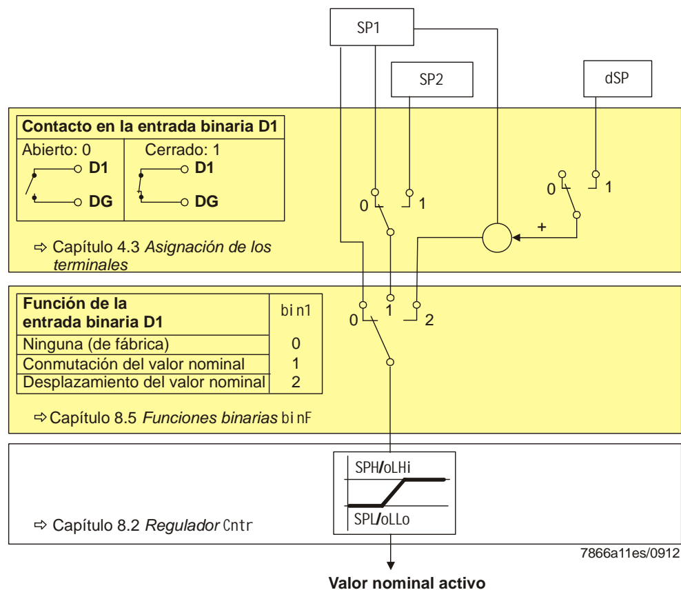
Figura 12: Conmutación o desplazamiento del valor nominal
