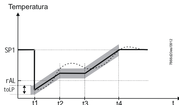
Figura 15: Protección contra choque térmico (TSS)
