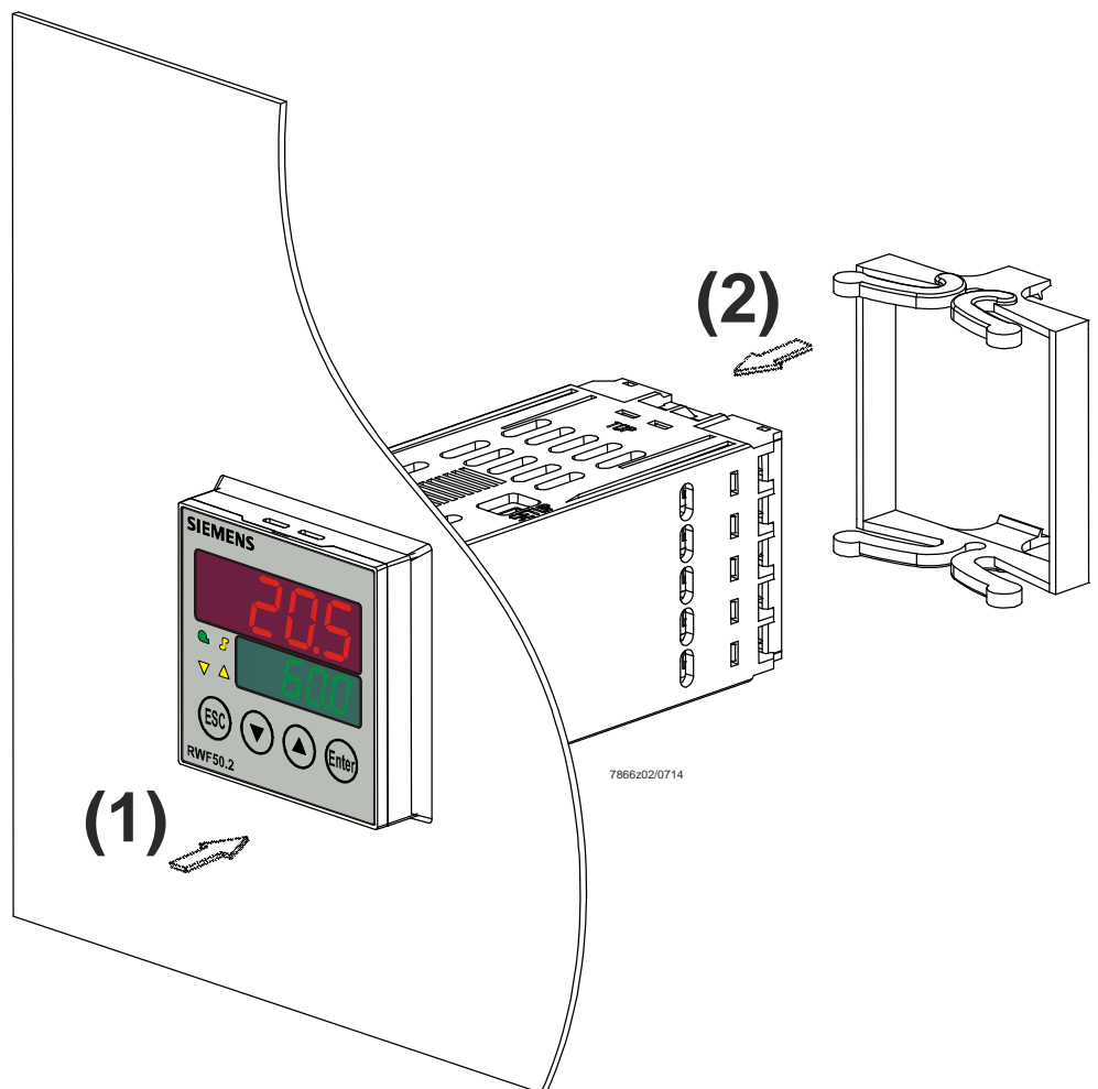
Figura 3: Montaje en abertura de cuadro de mando
