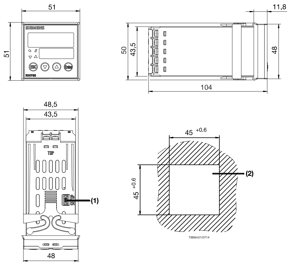
Figura 2: Dimensiones del RWF50
