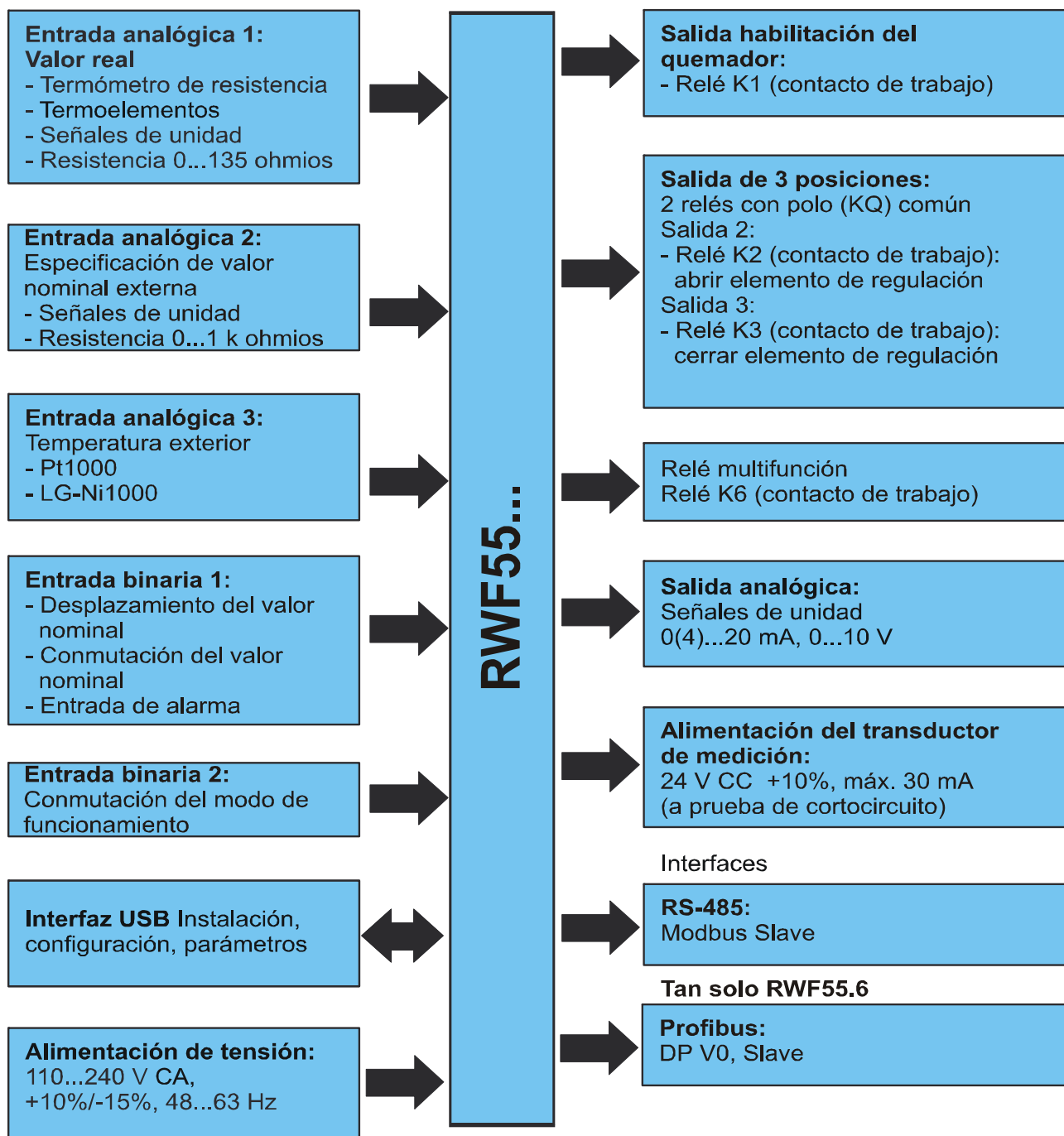
Figura 1: Estructura de bloques
