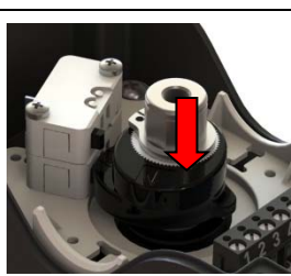
Abb. 4: Betätiger einstellen
