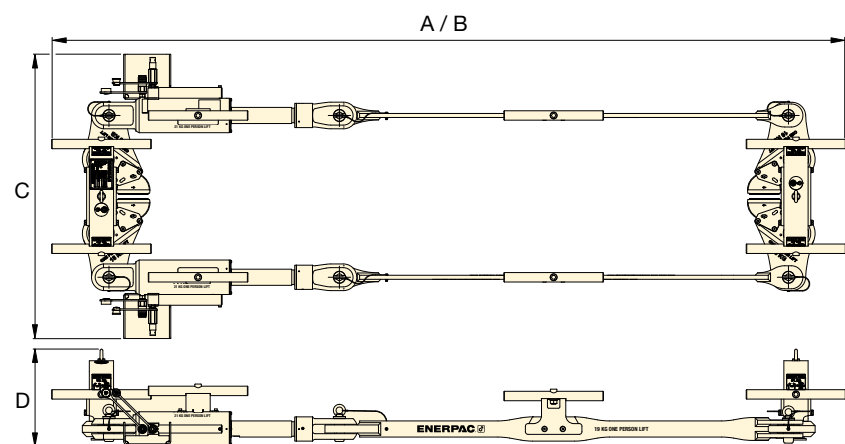
▲ Cadre de stockage et de transport RP70ATF avec stresser, pompe et possibilité de ranger en toute sécurité l'ensemble de tuyaux dans un espace de rangement verrouillable sous le cadre.
