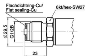
HDA 4X15 Einschraubzapfen/ Screwed end DIN EN 837-G1/2B
