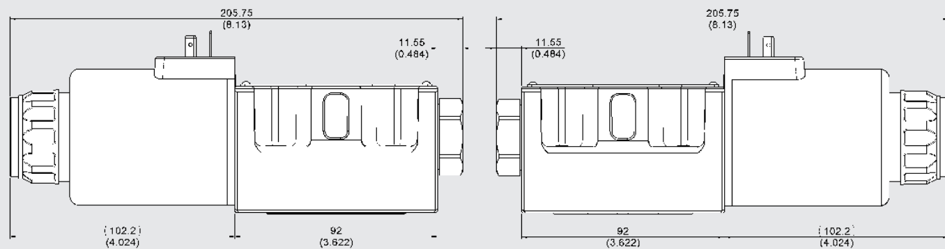
Ventil mit Magnet a
