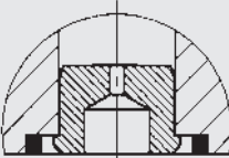
Einsteckblende Dient der Drosselung zu hoher Volumenströme, welche außerhalb der Betriebsgrenzen des Ventils liegen.
