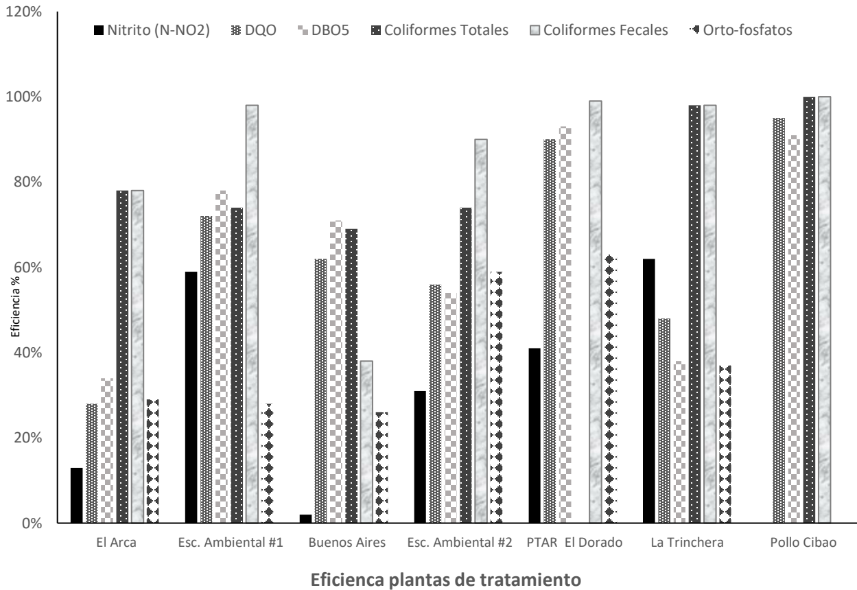
Figura 35. Eficiencia de las plantas de tratamiento de aguas residuales con Ingeniería Verde (El Autor, a partir de datos obtenidos en el proceso del estudio).
