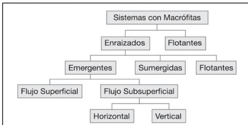
Figura 2. Esquema de clasificación de los sistemas de depuración con macrofita, según tipo de planta (Delgadillo et al., 2010).
