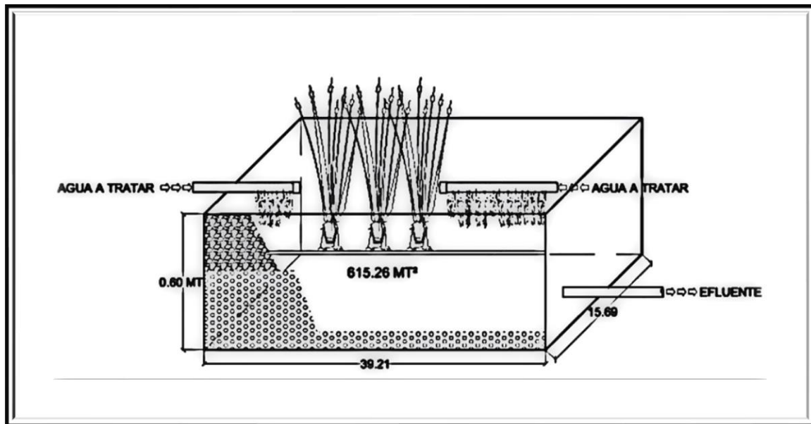
Figura 48. Diseño arquitectónico del humedal propuesto (elaboración propia).
