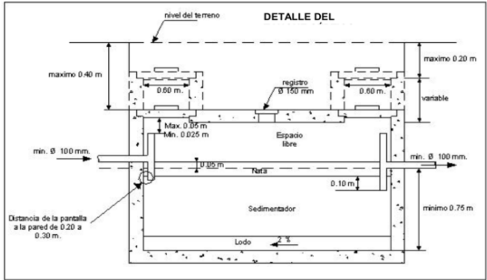
Figura 4. Tanque séptico cuadrado de dos compartimientos (OPS/CEPIS/05.163 UNATSABAR, 2005).
