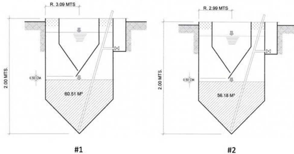
Figura 49. Tanque Imhoff -según Stier (Valter, 1989). Adaptado por el Autor de la tesis).
