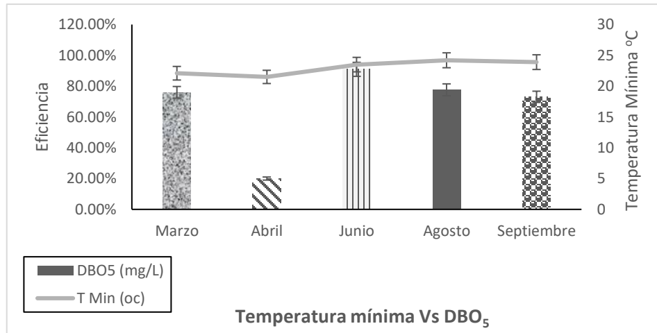
Figura 45.- Resultados de los efectos en la eficiencia de reducción de la DBO 5 con temperatura mínima (Plan Yaque, 2017 & INDRHI, 2018).
