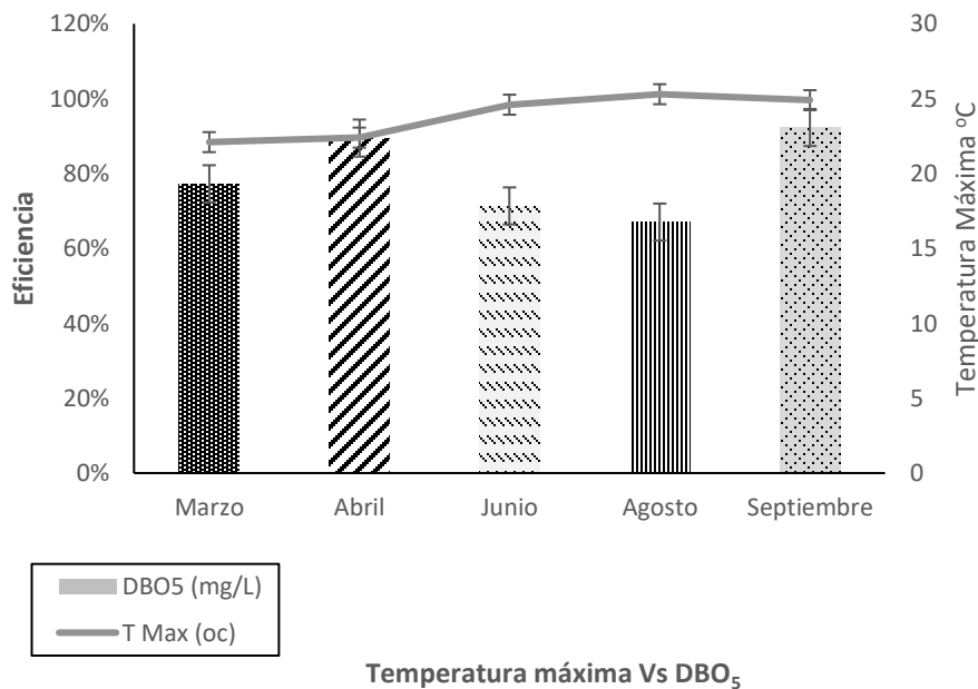
Figura 44.- Efectos en la eficiencia de reducción de la DBO5 con temperatura máxima (Plan Yaque 2017 & INDRHI 2018).
