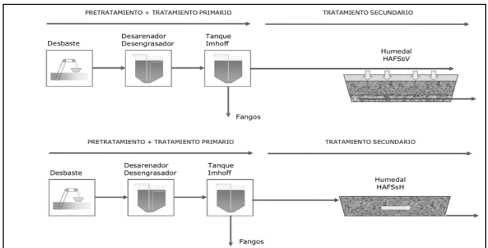
Figura 5. Operaciones unitarias tratamiento extensivo en humedales de flujo vertical (EPSAR, 2017).
