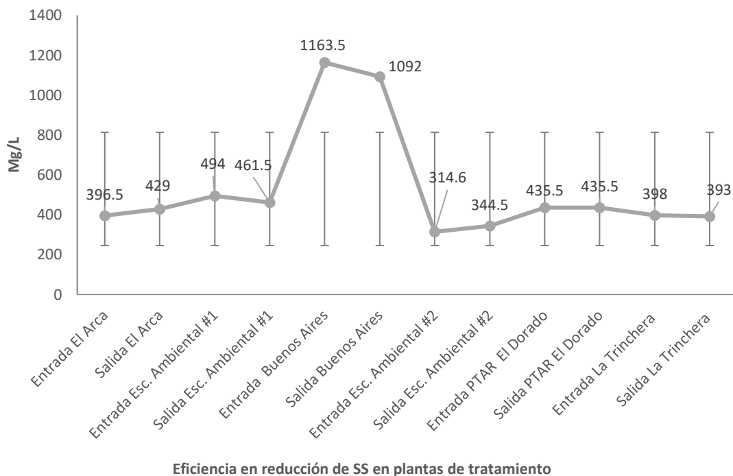
Figura 37. Resultados en la eficiencia de la reducción en total solidos disueltos (elaboración propia).
