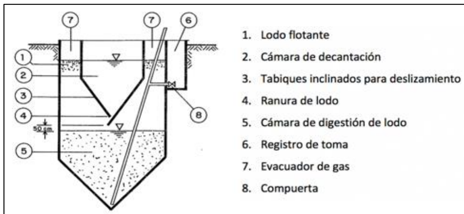
Figura 3. Tanque Imhoff, según Stier (Valter, 1989).
