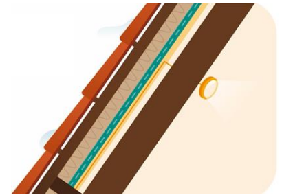
Dakisolatie met extra laag voor installaties
