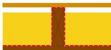
Dampdichte isolatie tussen balken
