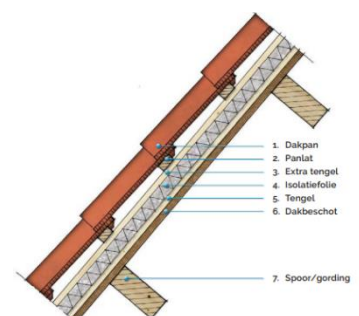
Isolatiefolie op het dakbeschoot
