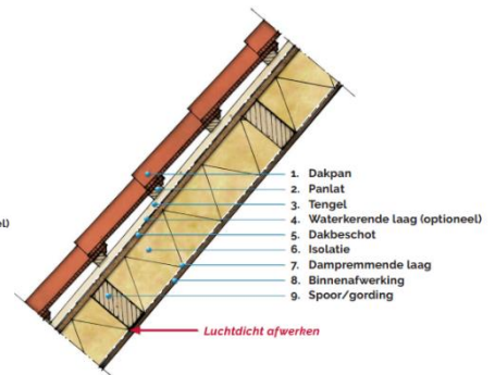
Isolatie tussen en afwerking over gordingen
