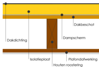
Warm dak isolatie
