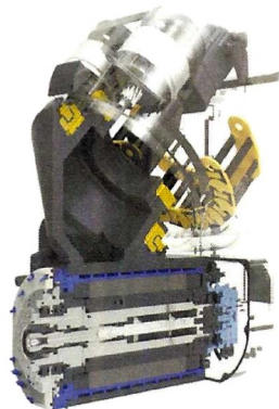
Innen liegender Kabelschlepp
