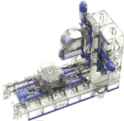
Temperierter Grundaufbau
