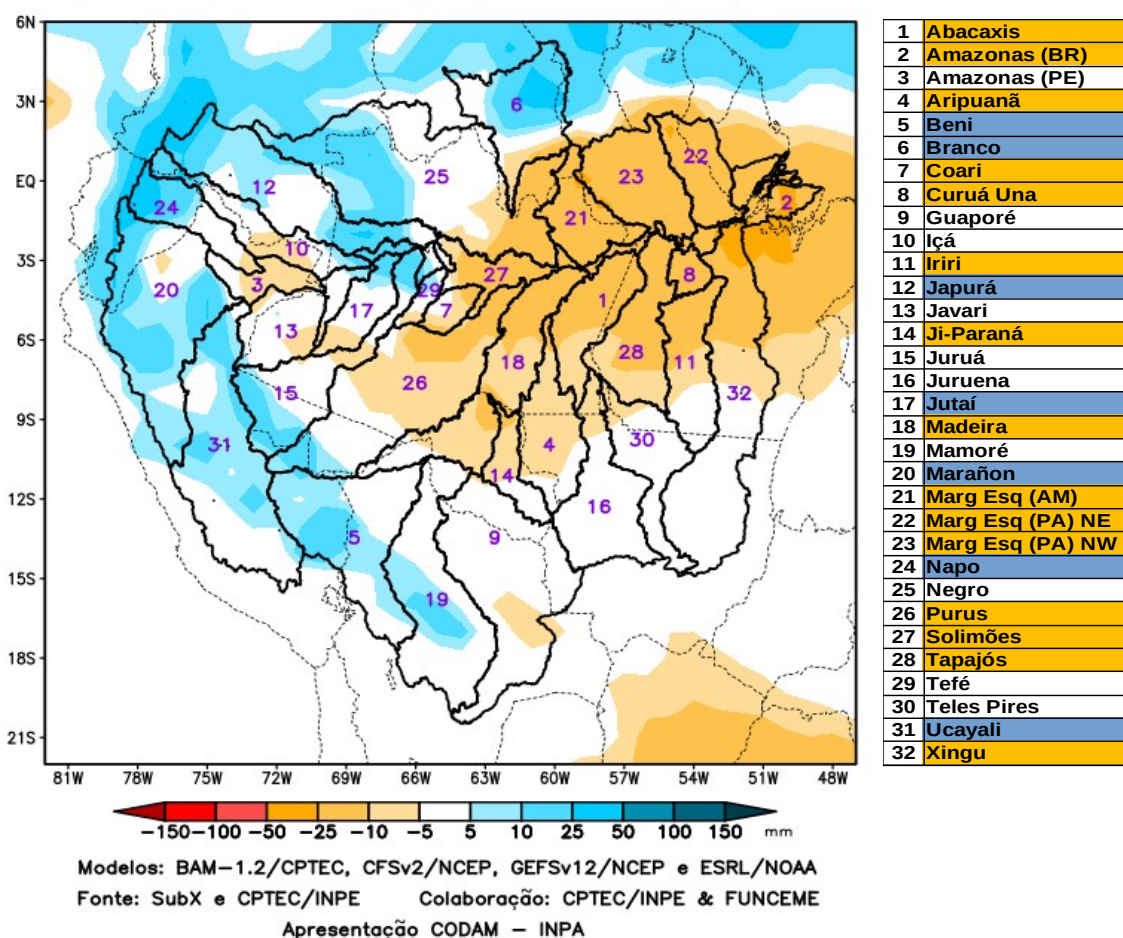
PREVISÃO SUBSAZONAL – MULTIMODELO CALIBRADO Anomalia (mm) de Precipitação Acumulada (07 Dias) Período: 12/06/2024 – 18/06/2024
