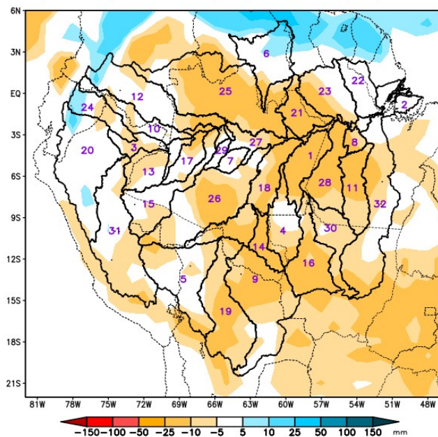
PREVISÃO SUBSAZONAL–MULTIMODELO CALIBRADO Anomalia (mm) de Precipitação Acumulada (07 Dias) Período: 09/11/2022 – 15/11/2022
