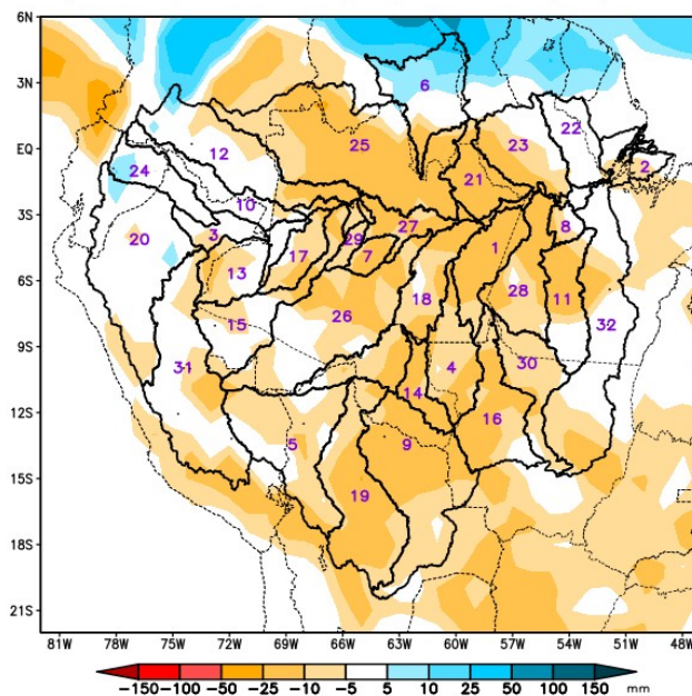
PREVISÃO SUBSAZONAL–MULTIMODELO CALIBRADO Anomalia (mm) de Precipitação Acumulada (14 Dias) Período: 09/11/2022 – 22/11/2022
