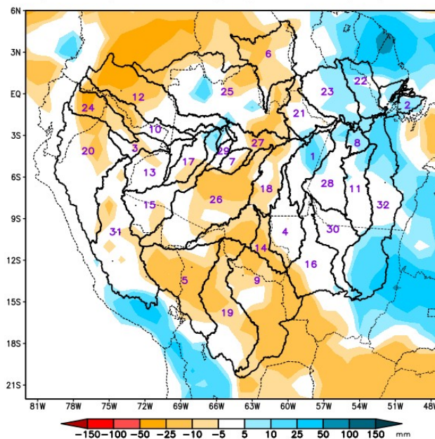
PREVISÃO SUBSAZONAL–MULTIMODELO CALIBRADO Anomalia (mm) de Precipitação Acumulada (14 Dias) Período: 07/12/2022 – 20/12/2022
