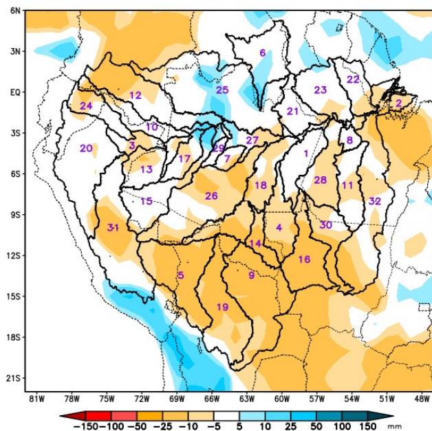
PREVISÃO SUBSAZONAL–MULTIMODELO CALIBRADO Anomalia (mm) de Precipitação Acumulada (07 Dias) Período: 07/12/2022 – 13/12/2022
