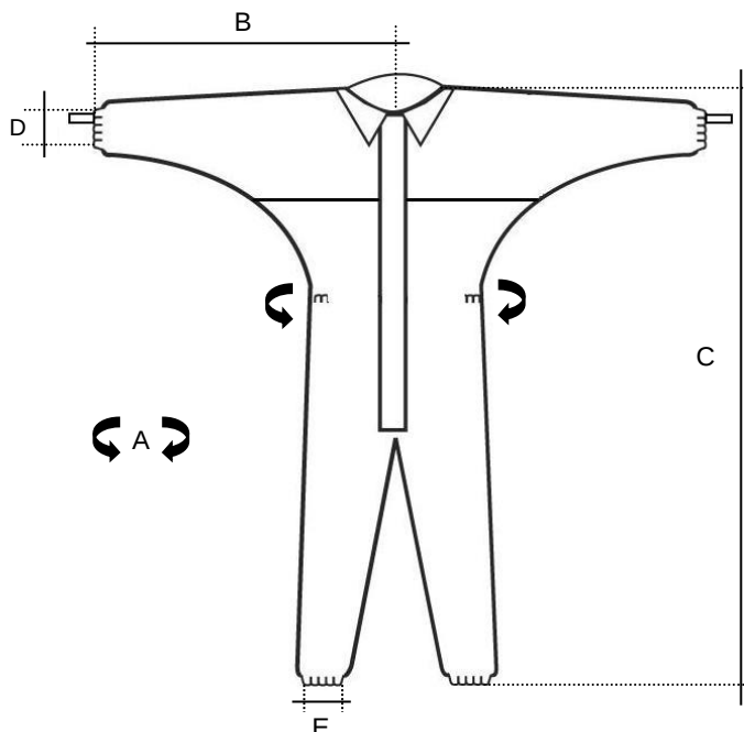
Fig. modèle et dimensions
