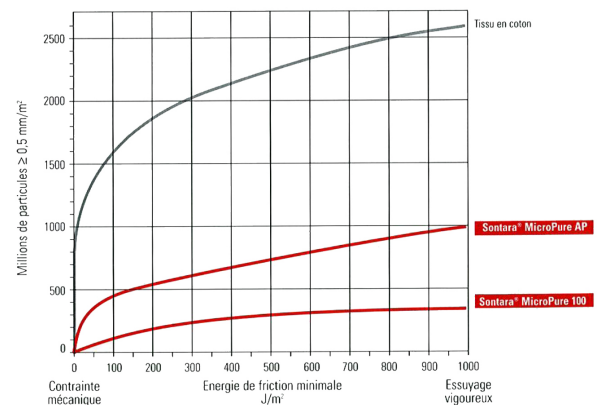
Courbes caractéristiques***
