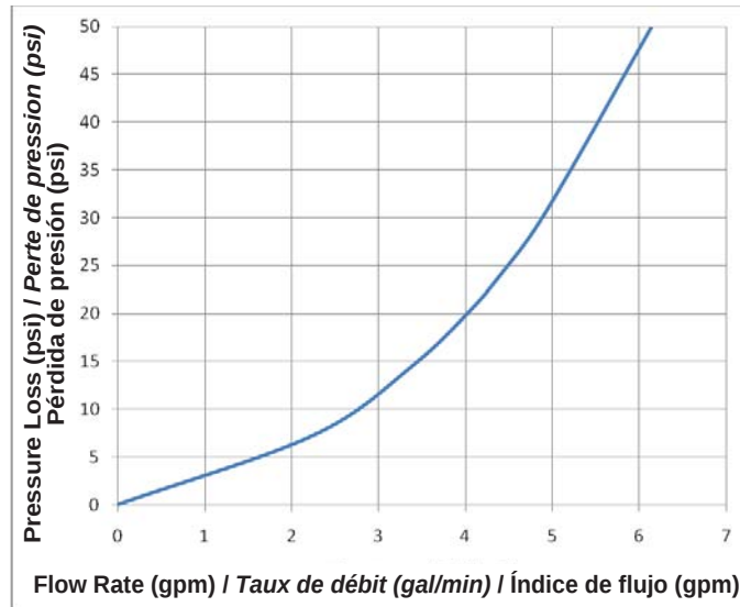
Diagram 2 - Flow Characteristics Diagramme 2 - Caractéristiques du débit Diagrama 2 - Características de flujo
