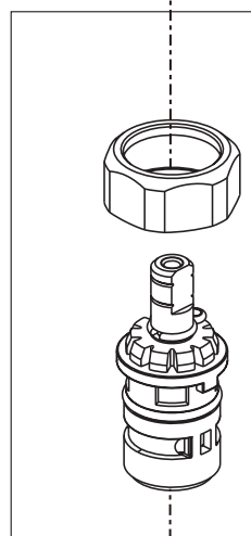
RP93981 Bonnet, Adapter & Valve Cartridge, Hot Side Bonete, Adaptador y Cartucho de la Válvula, Lado Chapeau, Adaptateur et Cartouche de soupape, Eau Chaude
