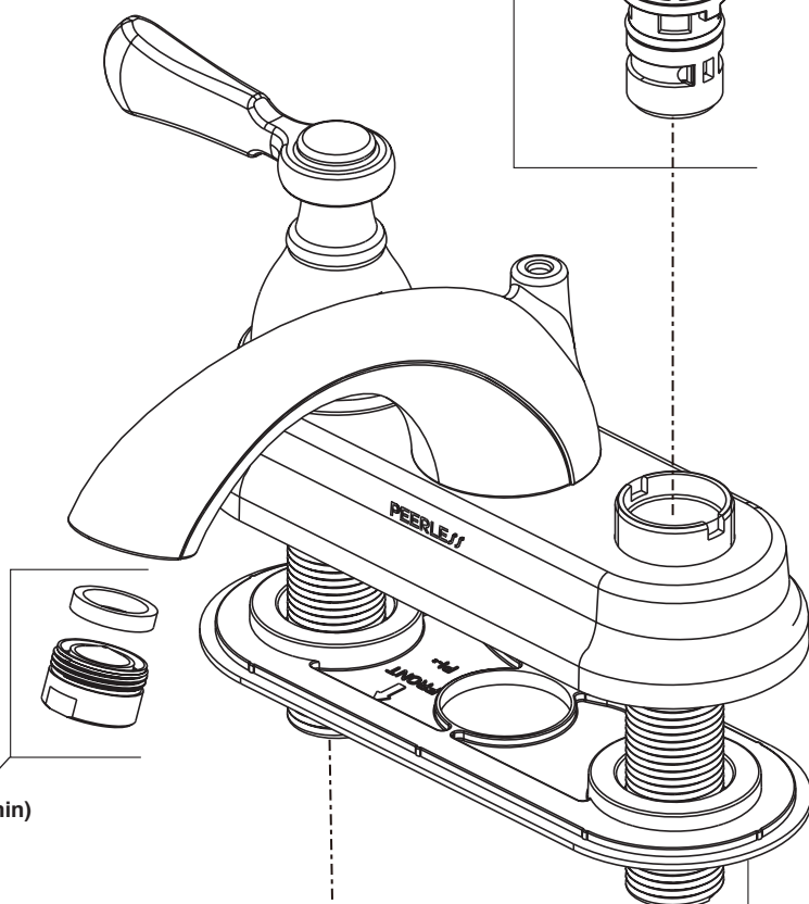
RP101332 Gasket & Baseplate Empaque y Placa de Base Joint et Plaque Definition
