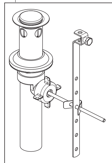
RP38958▲ 50/50 Pop-Up Assembly Less Lift Rod Ensamble del Desagüe Automático sin la barra para alzarlo Renvoi mécanique sans la tirette
