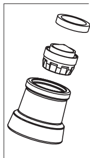
RP100275▲-1.0 1.0 GPM (3.8 L/min) Aerator Assembly Aireador Aérateur
