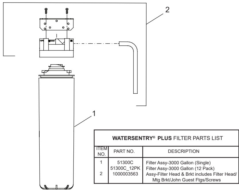
FIG. 12 Water Filter Exploded View Filtro de agua despiece Vue éclatée de l'eau filtre
