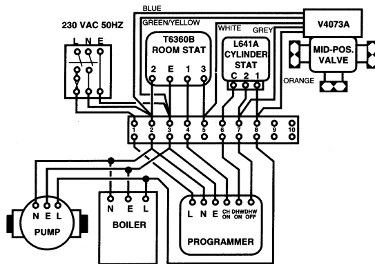
Fig. 4. Wiring Diagram
