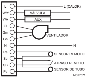
Fig. 12. Diagrama de cableado de dos tubos (calefacción o enfriamiento) con calefacción auxiliar y relevo manual (120 VCA/240 VCA/277 VCA en la ilustración).
