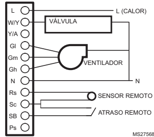
Fig. 9. Diagrama de cableado de dos tubos (calefacción o enfriamiento) con relevo manual (120 VCA/240 VCA/277 VCA en la ilustración).
