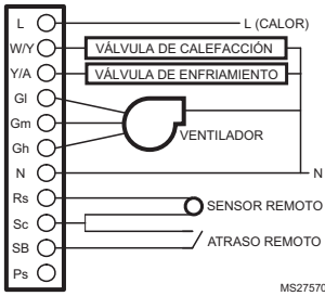
Fig. 11. Diagrama de cableado de cuatro tubos (calefacción y enfriamiento) con relevo manual/automático (120 VCA/240 VCA/277 VCA en la ilustración).
