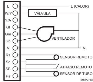
Fig. 10. Diagrama de cableado de dos tubos (calefacción o enfriamiento) con relevo automático (120 VCA/240 VCA/277 VCA en la ilustración).
