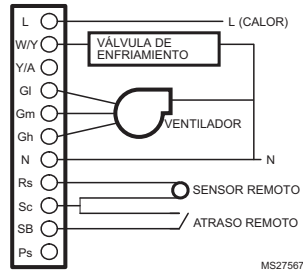
Fig. 8. Diagrama de cableado de dos tubos, solo enfriamiento (120 VCA/240 VCA/277 VCA en la ilustración).
