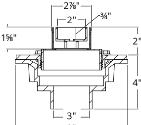
S-TIFAS 99
