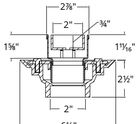
S-TIFAS 65
