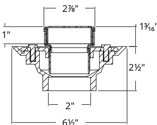
S-DGAS 65, S-AS 65
