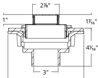
S-DGAS 99, S-AS 99
