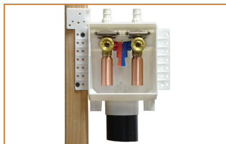
1 Box - To Stud
