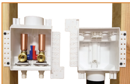
2 Box - Separate Stud Same Bay
