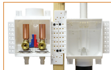
2 Box - Straddle Stud
