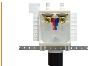
1 Box - Inside Stud Bay Hyco Strap
