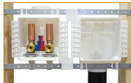
2 Box - Inside Stud Bay Hyco Strap
