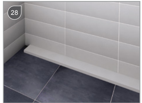
Vloortegels plaatsen / Fixation of the floor tiles / Poser le carrelage au sol contre le guide de pose en polystyrène / Bodenfliesen bis an das Styropor Rinnen Innenteil ankleben
