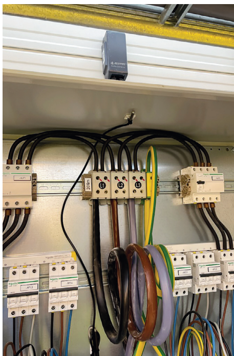
Temperaturføleren ses i toppen av skapet.
