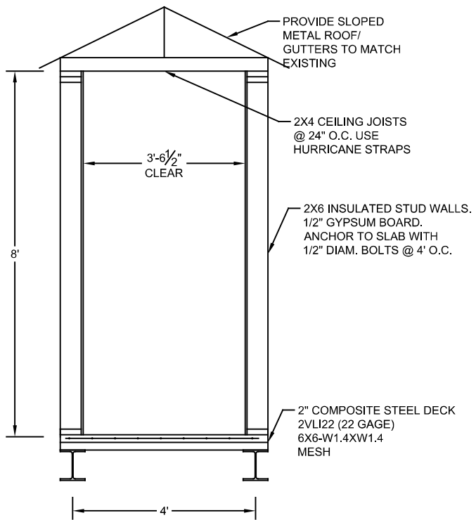
1 SECTION S2 SCALE: 1" = 1'-0"
