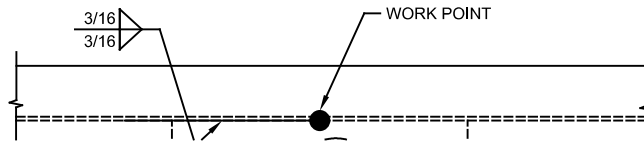
1 SECTION S2 SCALE: 1" = 1'-0"
