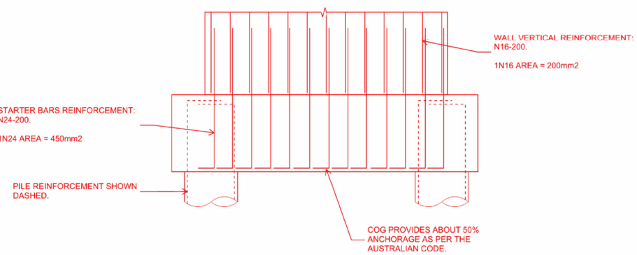
W1 ELEVATION
