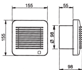
Målskitse EDM 100:
