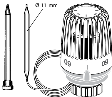
Med følerlomme (tilbehør) som dykrørsføler
