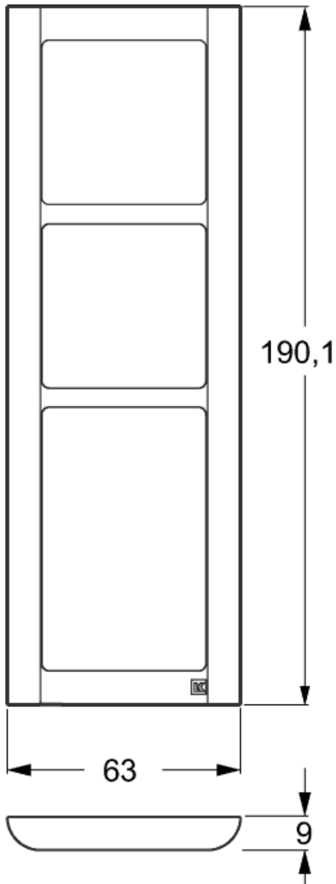
Målskitse
