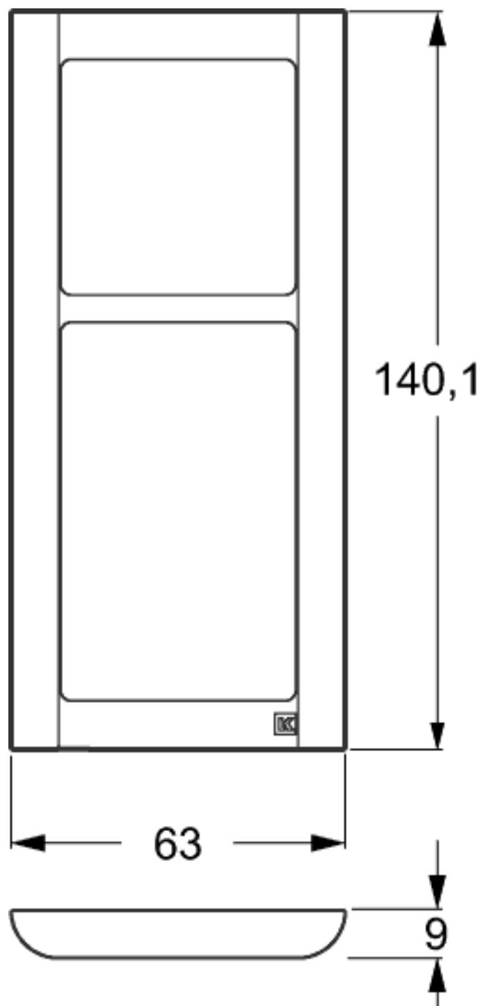
Målskitse
