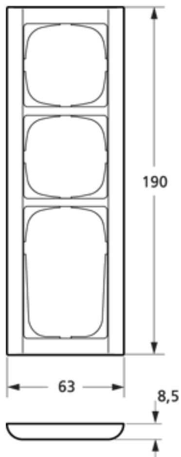
Målskitse
