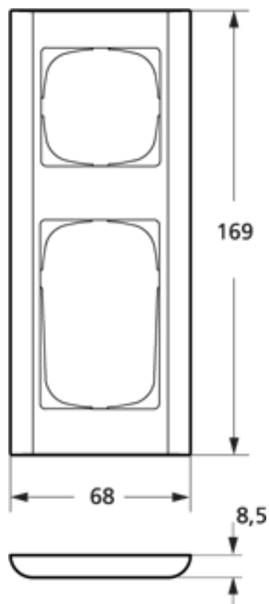
Målskitse
