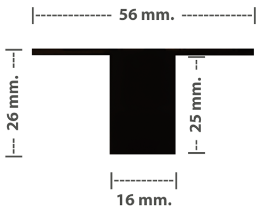
Planforsænket lysskinne:
