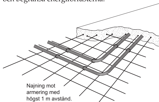
Klamring mot armering. Najning mot armering med högst 1 m avstånd.
