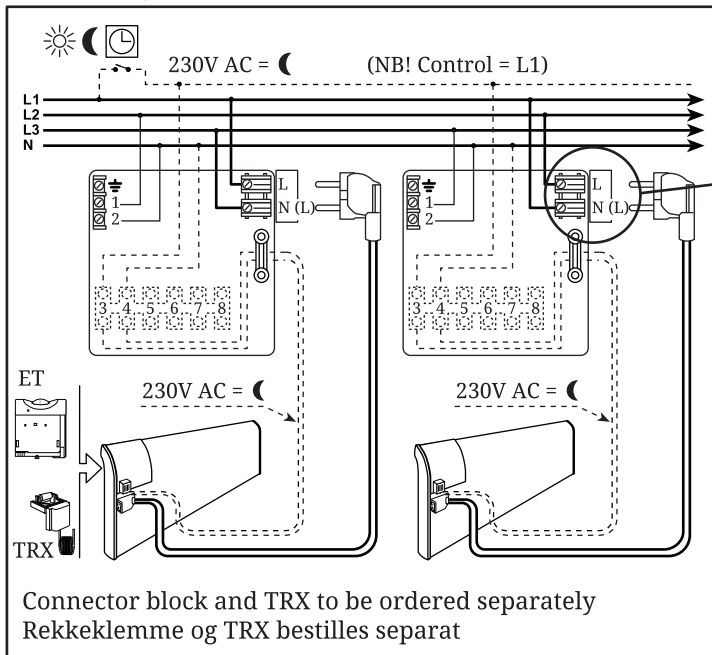
230 volt diagram
