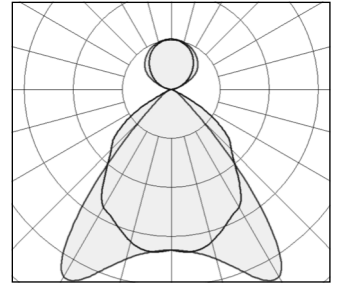
AREL med mat reflektor afskærmning, med oplys
