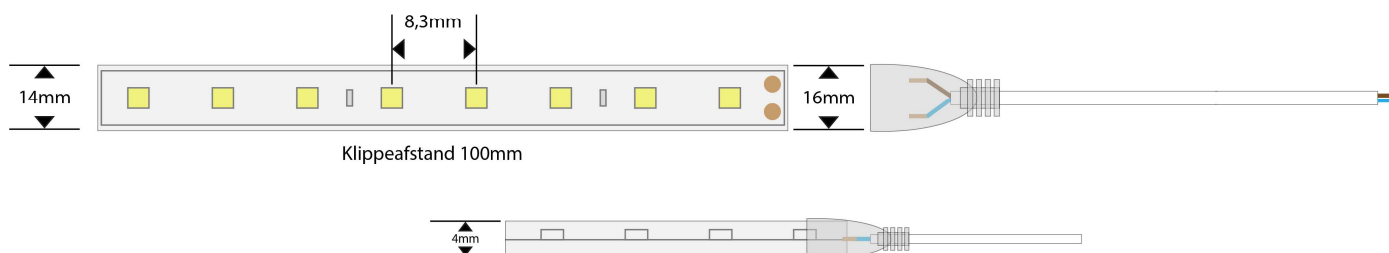
Målskitse for 230V 10cm 10W Led Strip
